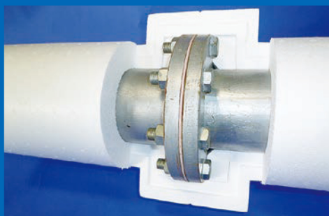
ダイヤフランジカバーは、独立体の形状のために直管部との接続性に優れ、後施工やメンテナンスが容易に出来ます。
